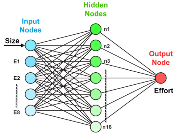
Fig. 9. MLP model.
